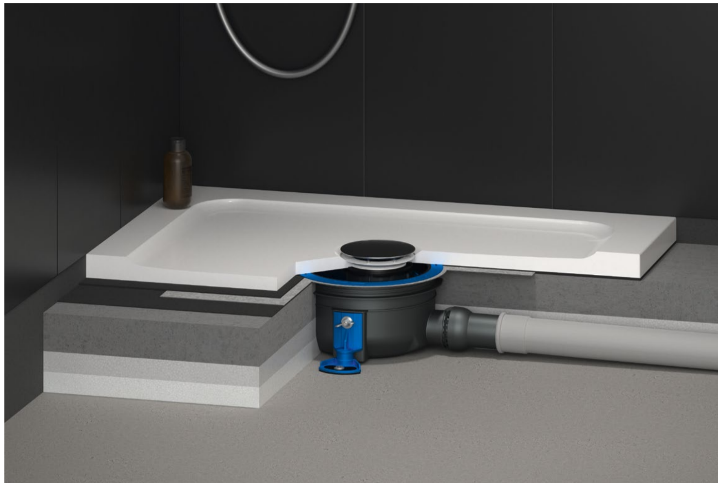
Duschwannenablauf ORIO DallBox, abgebildet mit Abdeckhaube Edelstahl
