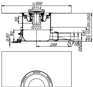
Duschwannenablauf ORIO DallBox, Abdeckhaube Edelstahl
