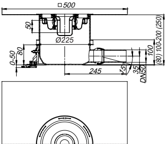
Ablaufgehäuse ORIO DallBox (ohne Abdeckhaube*)
